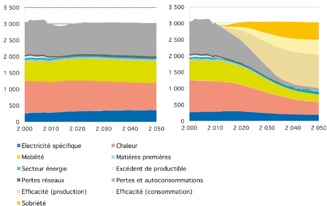
■ Evolution comparée des consommations énergétiques finales par usages entre le scénario tendanciel et le scénario négaWatt (en TWh)
